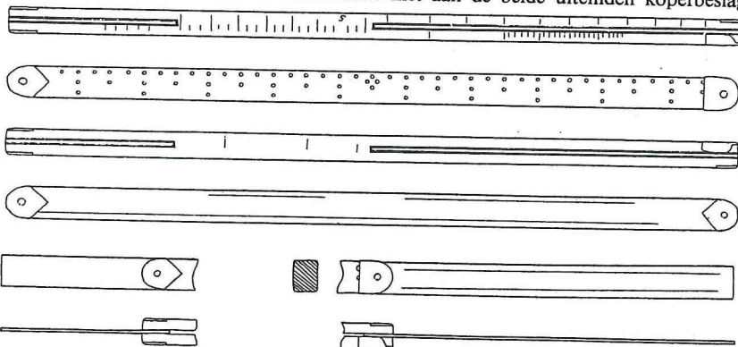
Afb. 22. Vollemolen. « Mechelse voet ». Tekening F. De Buyser.
