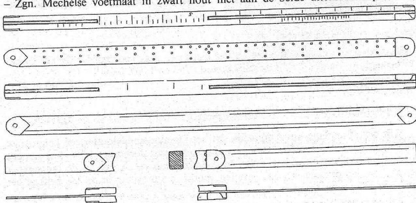
Afb. 22. Vollemolen. « Mechelse voet ». Tekening F. De Buyser.
